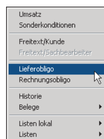
Popup-Menü Kunde
