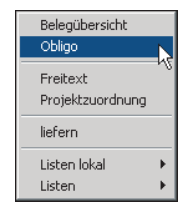
Popup-Menü EK
