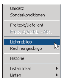
Popup-Menü Lieferant
