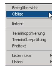
Popup-Menü VK
